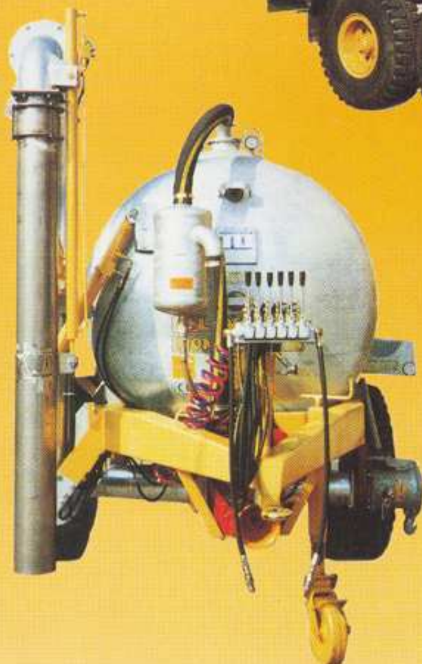
CARROBOTTE con braccio comandato a distanza
